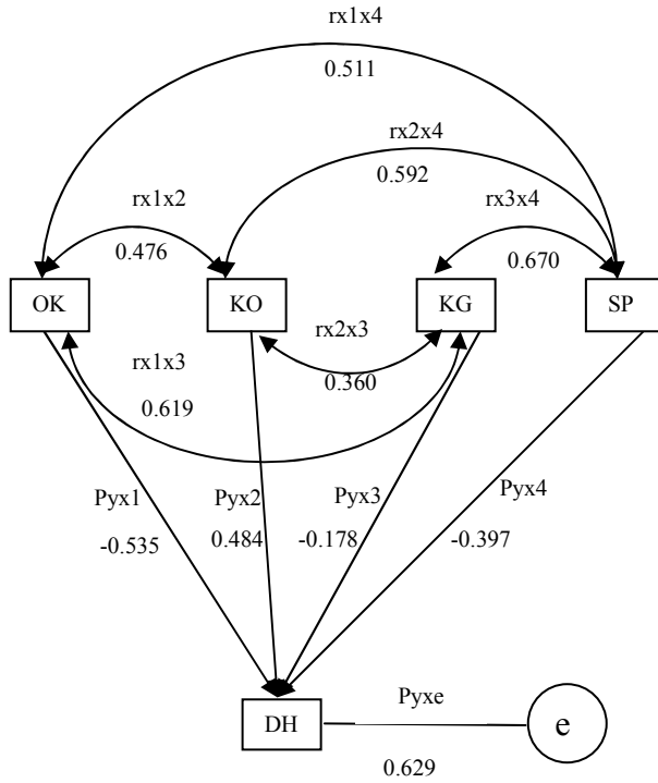
Şekil 2. Çıktı Path Diyagramı
